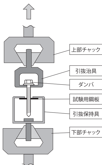
単体引抜保持力試験方法
